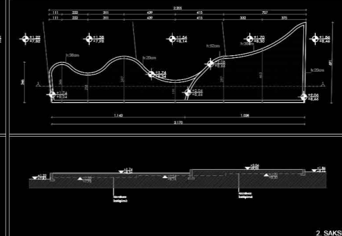
MEYDAN MU 05 BETONARME SAKSI PLANI-2 1/50 MEHMETÇİK PARKI MEYDAN TASARIMI 01.10.2024
